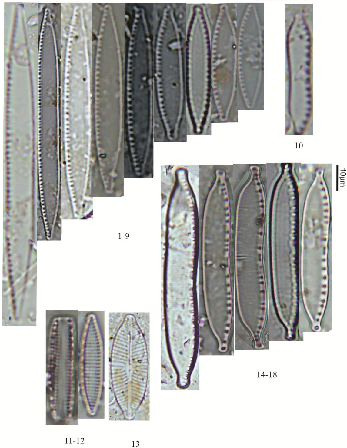
1-9 Synedra palea ; 10 Nitzschia brevissima ; 11-12 Nitzschia amphibia (11 VV); (12 VP); 13 Geissleria neosubtropica ; 14-18 Eunotia amphioxys .
